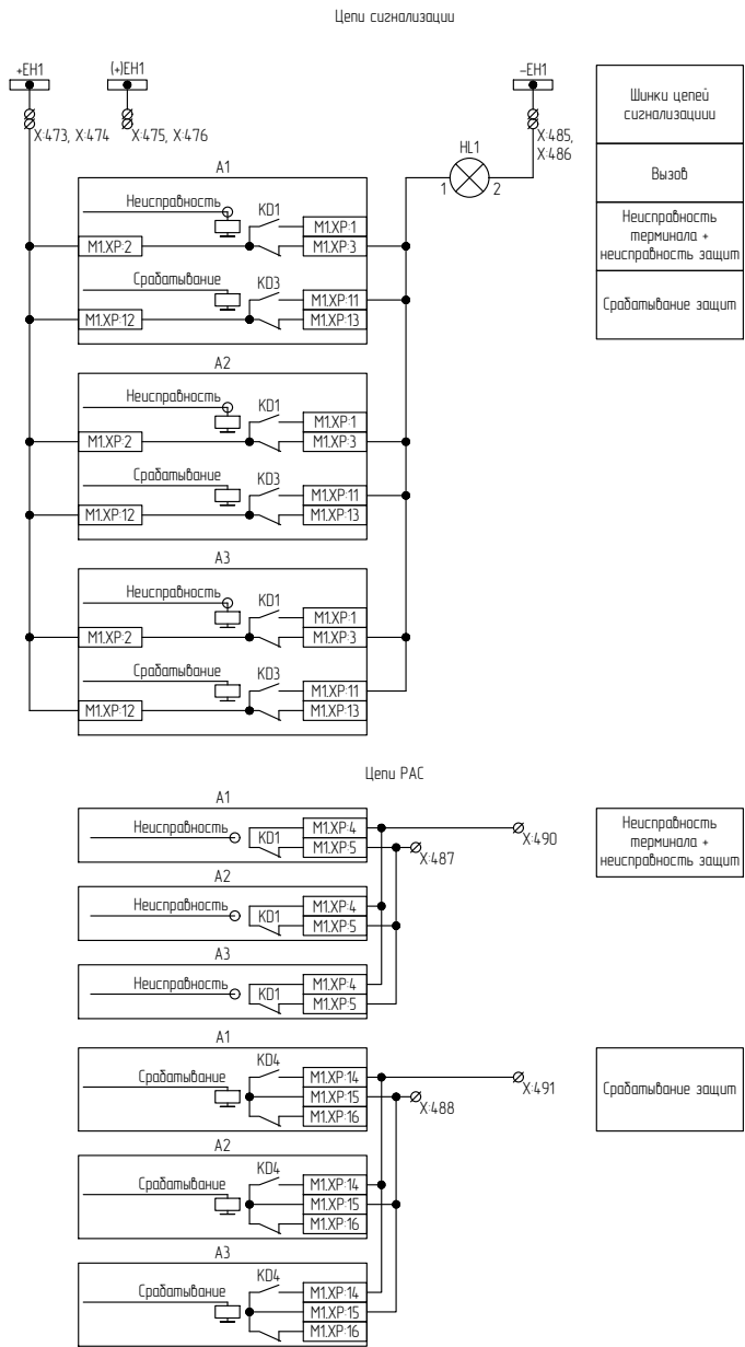
Рисунок В.18 – Схема электрическая принципиальная (часть 18)
